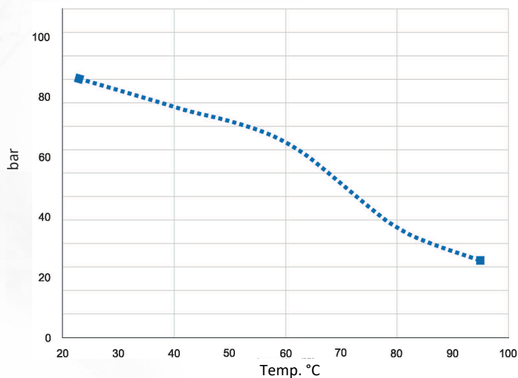
Zależność temperatury od ciśnienia/ Dependence of temperature on pressure
